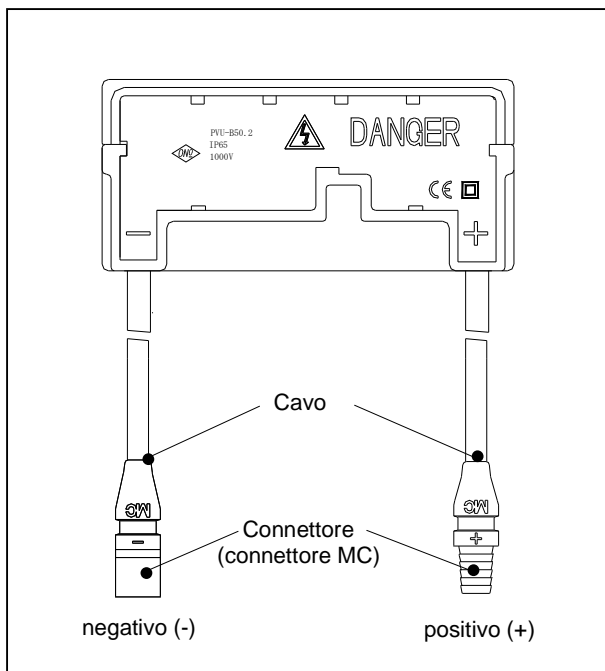
Figura 3: Aspetto della scatola di giunzione
