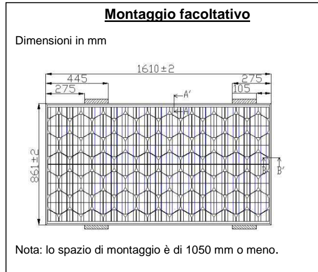
Figura 2-3: Montaggio facoltativo
