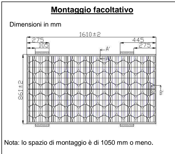
Figura 2-2: Montaggio facoltativo
