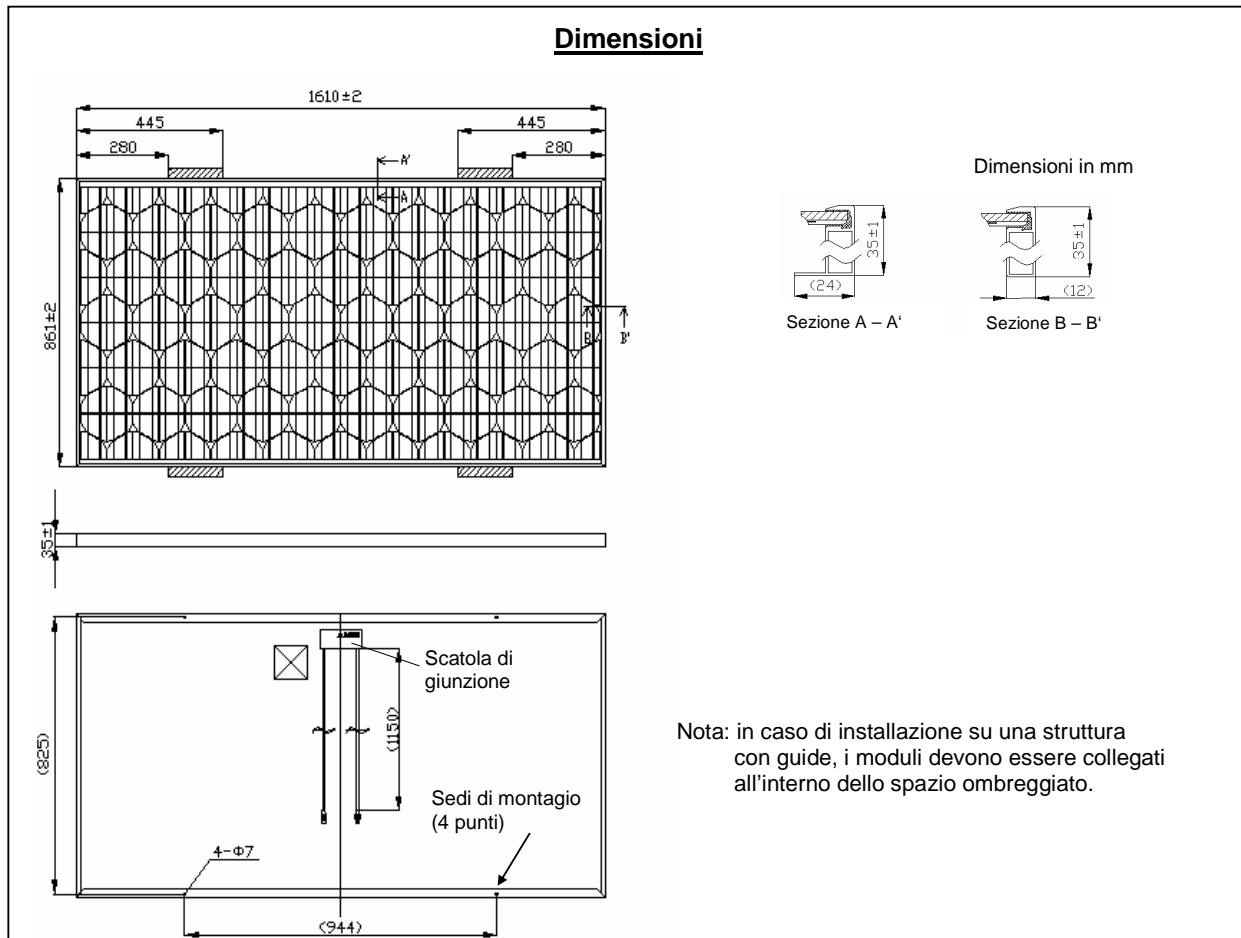
Figura 2-1: Dimensioni
