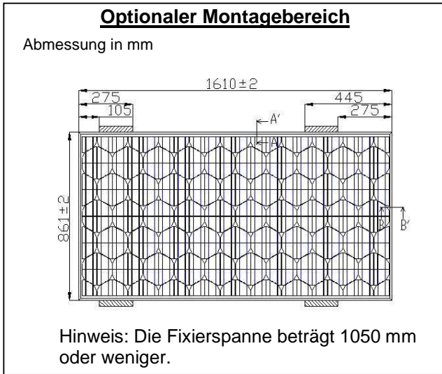
Abb. 2-2: Optionaler Montagebereich
