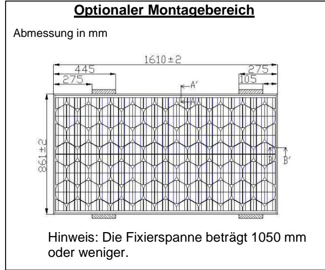
Abb. 2-3: Optionaler Montagebereich
