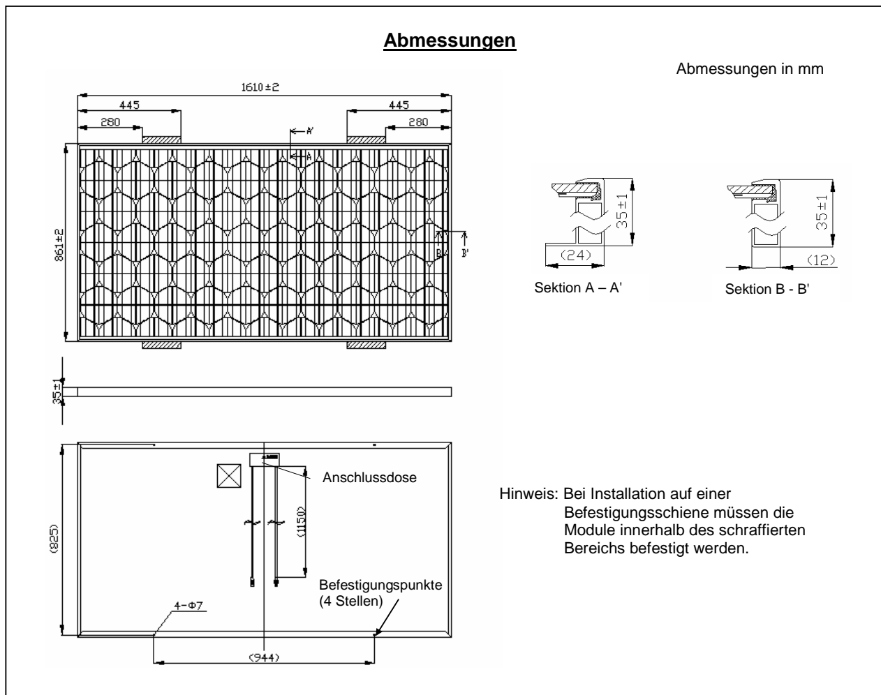
Abb. 2-1: Abmessungen
